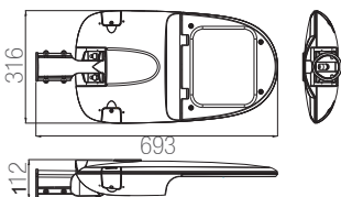
Tamaño de luminarias (mm) desde 40w hasta 120w
