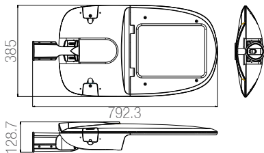
Tamaño de luminarias (mm) desde 150w hasta 220w
