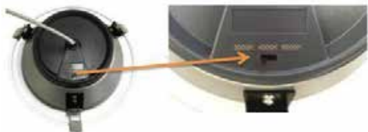
SWITCH PARA CAMBIO DE TEMPERATURA 3000K - 4000K - 6000K
